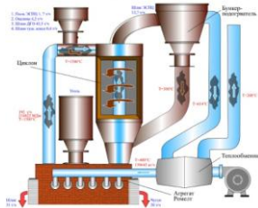
Металлургический комплекс "Энергетри - печь Ванюкова - пикет"
