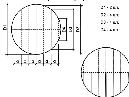
Рисунок 17. Развертка сферы с 6 сегментами
