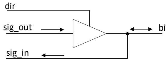
Рисунок 2.2 – Двухнаправленный порт
