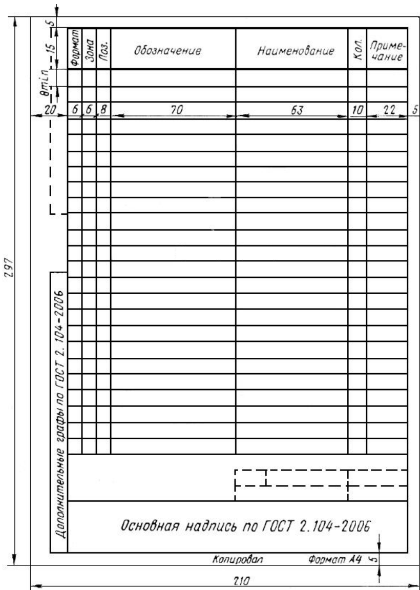
Рис. 3.5. Общая форма спецификации по ГОСТ 2.106-96 ЕСКД
