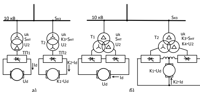
Рис. 1.1. Схемы присоединения ТП к сети 10 кВ однофазных(а) и двухфазных(б)
