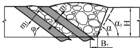
Рис. 5.1 – Параметры залегания пластов на уступе, разрабатываемых по схеме с проходкой разрезной траншеи со стороны кровли верхнего пласта: H – высота вскрышного уступа, м; \phi – угол залегания пластов, град; m_1 и m_2 – соответственно мощность нижнего и верхнего пласта свиты, м; M – мощность между-пластья, м; B_T – ширина разрезной траншеи по дну ( B_T = 3\text{м} ); \alpha_y , \alpha – соответственно устойчивый и рабочий углы откоса вскрышного уступа, град
