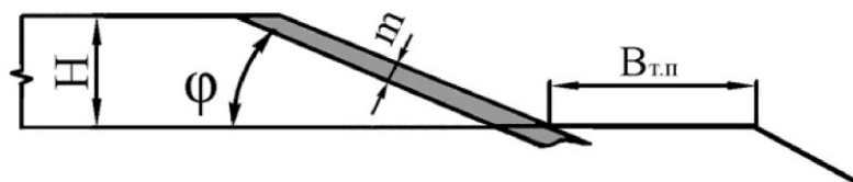
Рис. 6.1 – Параметры залегания наклонного пласта: H – высота вскрышного уступа, м; φ – угол залегания пласта, град; m – мощность пласта, м; В т.п – ширина транспортной площадки, м
