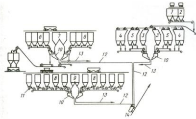
Рис. 6. Схема шихтоподдачи доменной печи "Alpanda" объемом 2032 м 3 . 1 – бункера окатышей; 2, 3 – бункера известняка; 4 – бункера агломерата и руды; 5 – бункера окатышей и руды; 6, 7 – бункера кокша; 8 – бункера дозавок; 9 – бункер скрала; 10 – весовые воронки; 11–13 – ленточные весы; 14 – скрап.
