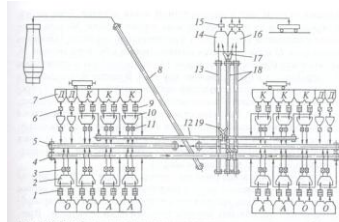
Рис. 5.70. Схема конвейерной шихтоподдачи доменной печи объемом 5000 м 3 .
