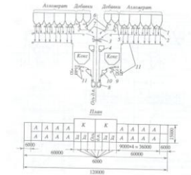
Рис. 5.69. Схема трансформаторной шихтоподдачи к скатам доменной печи объемом 3200 м 3 . 1 – флюид агломерата; 2 – конвейер агломерата; 3 – вертикальный лоток; 4, 6, 10 – весовые весы; 5 – ленточный конвейер; 7 – конвейер руды; 8 – конвейер кокша; 9 – конвейер кокша; 11 – конвейер кокша; 12 – конвейер кокша; 13 – конвейер кокша; 14 – конвейер кокша.
