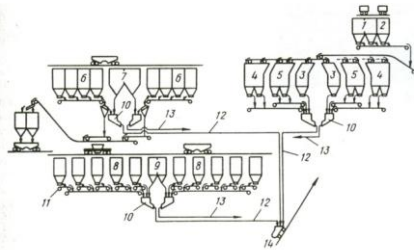
Рис. 6. Схема шихтоподачи доменной печи "Амалда" объемом 2032 м 3 . 1 – бункера окатышей; 2, 3 – бункера известняка; 4 – бункера агломерата и руды; 5 – бункера окатышей и руды; 6, 7 – бункера кокса; 8 – бункера добавок; 9 – бункер скрапа; 10 – весовые воронки; 11–13 – ленточные веса; 14 – скип
