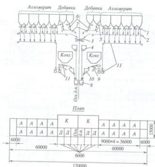
Рис. 5.69. Схема транспортной шихтоподачи к скипам доменной печи объемом 3200 м 3 . 1 – громот агломерата; 2 – конвейер агломерата; 3 – перекалный лоток; 4, 6, 10 – воронка-леса; 5 – питатель добавок; 7 – конвейер добавок; 8 – скип; 9 – громот кокса; 11 – конвейер уборки мезели.
