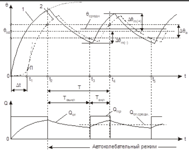
График двухпозиционного регулирования при двухёмкостном объекте с самовыравниванием и переходным запаздыванием: 1 - график изменения температуры греющей среды; 2 - график изменения температуры датчика температуры изделия
