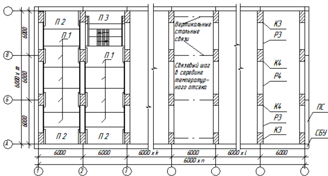
Рисунок П.1. - Схема плана с сеткой колонн 6×6 м (вариант 1)
