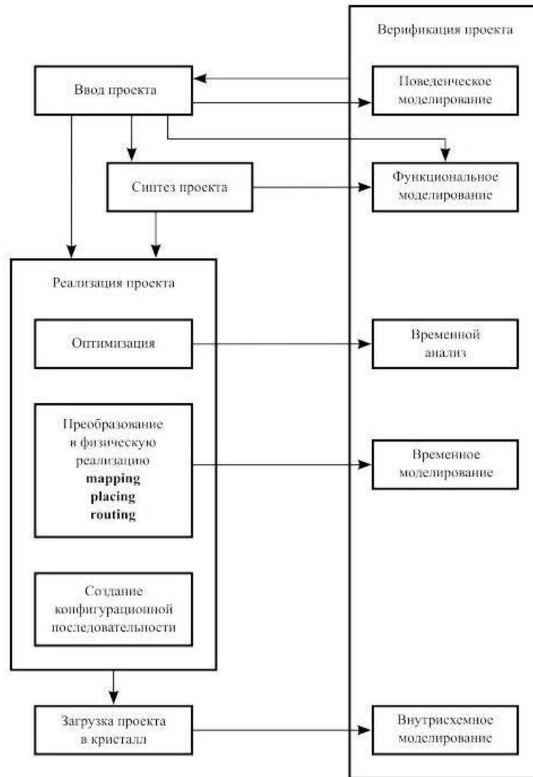
Рисунок 2 - Обобщенная схема проектирования цифровых устройств в САПР WebPAC
