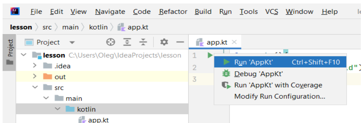
Рис. 5. Запуск программы
