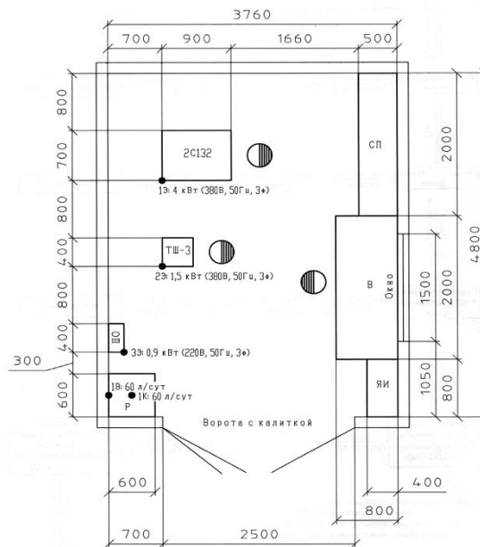
Компоновка мастерской
