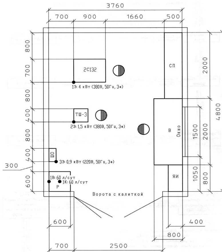
Рисунок 6.3 – Компоновка мастерской
