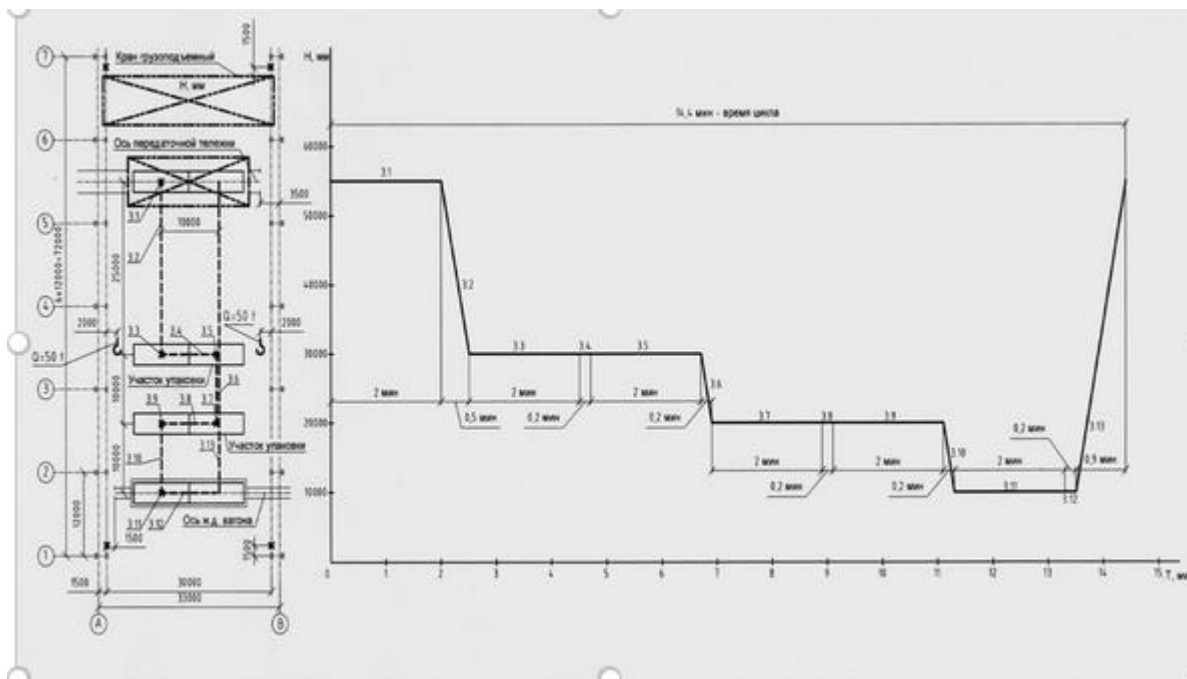
Рисунок 6.2 – Циклограмма работы грузоподъемного крана
