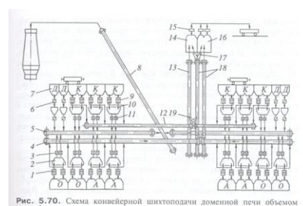
Рис. 5.70. Схема конвейерной шихтоподдачи доменной печи объемом 5000 м 3
