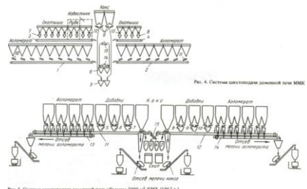
Рис. 5. Система шихтоподдачи доменной печи объемом 2000 м 3 КМЗ (1962 г.)
