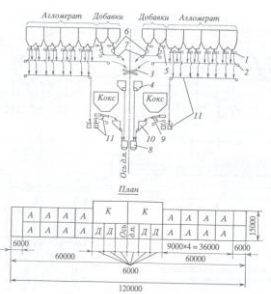
Рис. 5.69. Схема транспортной шихтоподдачи к скипам доменной печи объемом 2000 м 3 . 1 – грохот алмазита; 2 – конвейер алмазита; 3 – перекидной лоток; 4, 6, 10 – воронка-весы; 5 – инертиль добавок; 7 – конвейер добавок; 8 – скип; 9 – грохот кокса; 11 – конвейер борна мелкого
