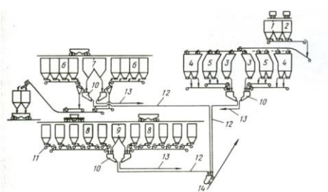
Рис. 6. Схема шихтоподдачи доменной печи "Аманды" объемом 2032 м 3 . 1-бункера окатышей; 2,3-бункера известняка; 4-бункера агломерата и руды; 5-бункера окатышей и руды; 6,7-бункера кокса; 8-бункера добавок; 9-бункер скрапа; 10-весовые воронки; 11-13-ленточные весы; 14-скип
