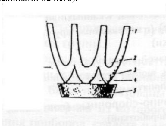
а -крапановая часть; б -оконная часть; 1 -крапан; 2 -люфт; 3 -бок; 4 -окно; 5 -рант
