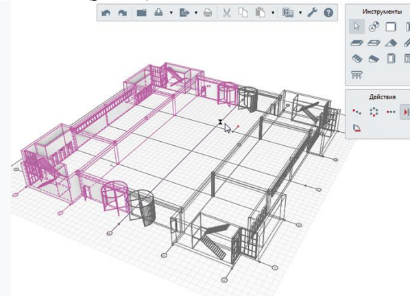
Рис. 5. Применяем симметрию
