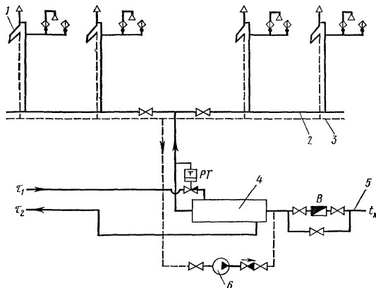
1 — полотенцесушитель; 2, 3 — подающая и циркуляционная линии; 4 — секционный водонагреватель; 5 — водопровод; 6 — циркуляционный насос; В — водомер
