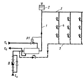
1 — подающий стояк; 2 — воздухоотделитель; 3 — верхний розлив; 4 — разборный стояк; 5 — циркуляционная линия; В — водомер на линии водопроводной воды
