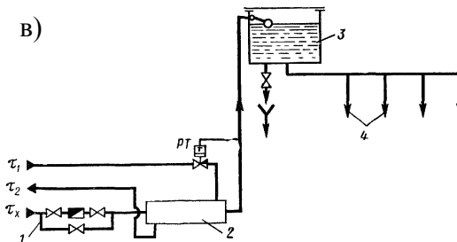
1 — водопроводная вода; 2 — секционный водонагреватель; 3 — верхний бак-аккумулятор с поплавковым краном; 4 — к водоразборным приборам; РТ — регулятор температуры
