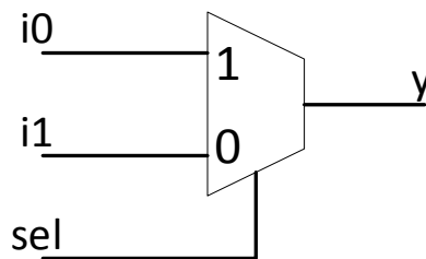
Рисунок 2.3 – Схема мультиплекса 2 в 1
