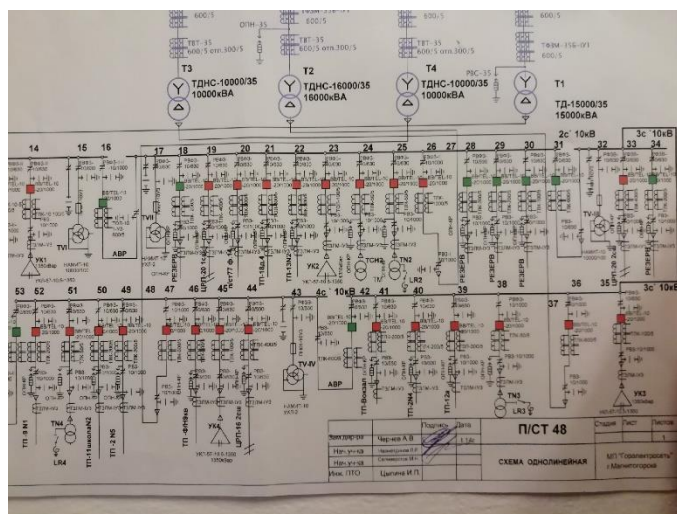
Рис 20 – Однолинейная схема
