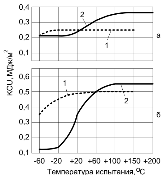
Рис. Вязкость сталей 6XС (1) и 6ХВ2С (2) в зависимости от температуры испытания: а – закалка на мелкое зерно и отпуск при 250 °С; б – изотермическая закалка при 250 °С
