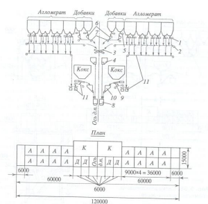
Рис. 5.69. Схема транспортной шихтоподдачи к склидам доменной печи объемом 2000 м 3 . 1 – грохот агломерата; 2 – конвейер агломерата; 3 – шредный ленточ; 4, 6, 10 – воронка-весы; 5 – питатель лобовок; 7 – конвейер лобовок; 8 – скин; 9 – грохот кокса; 11 – конвейер обрешетки
