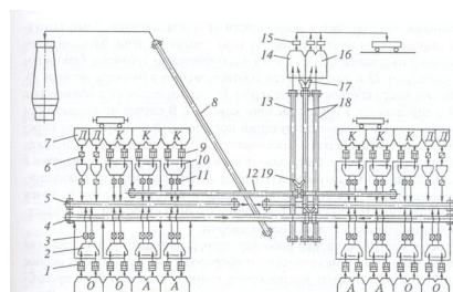
Рис. 5.70. Схема конвейерной шихтоподдачи доменной печи объемом 5000 м 3 .
