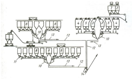
Рис. 6. Схема шихтоподачи доменной печи "Atapala" объемом 2032 м³: 1-бункера окатышей; 2,3-бункера известняка; 4-бункера агломерата и руды; 5-бункера окатышей и руды; 6,7-бункера кокша; 8-бункера доломитов; 9-бункер скрала; 10-весовые воронки; 11-13-ленточные весы; 14-скал
