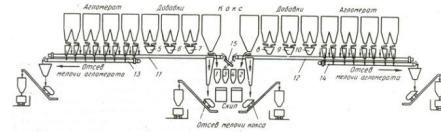
Рис. 5. Система шихтоподачи доменной печи объемом 2000 м³ КМЗ (1962 г.)
