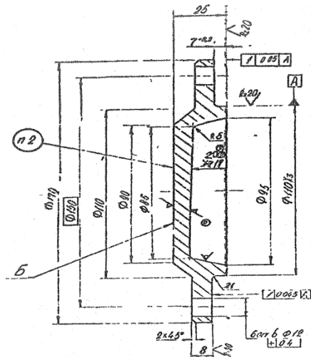
Рис. 1. – Пример чертежа литого изделия
