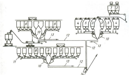
Рис. 6. Схема шихтоподдачи доменной печи "Amalinda" объемом 2032 м 3 . 1 – бункера окатышей; 2,3 – бункера известняка; 4 – бункера агломерата и руды; 5 – бункера окатышей и руды; 6,7 – бункера железца; 8 – бункера лобовок; 9 – бункер скрала; 10 – весовые воронки; 11–13 – ленточные весы; 14 – скли
