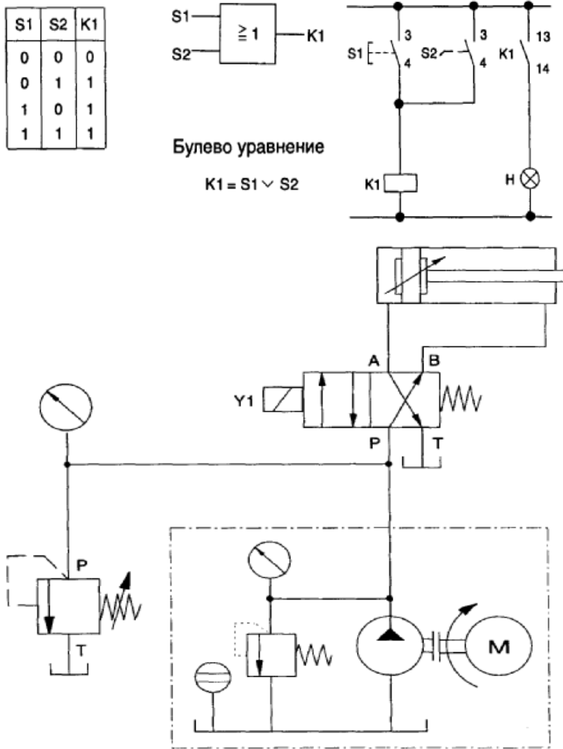
1 электрическая схема
