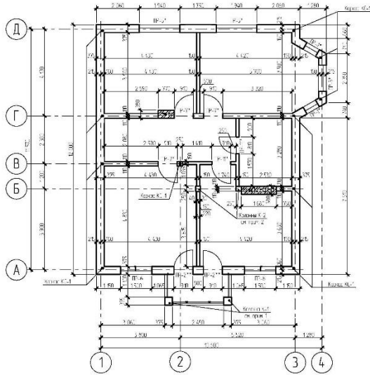
Кладочный план 2 этажа
