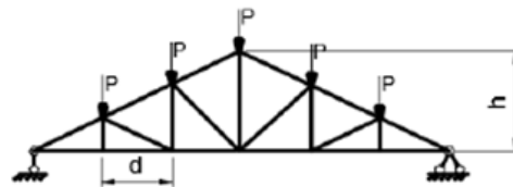
Рисунок 1 – Расчетная схема фермы
