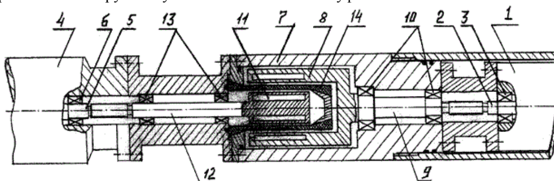
14.2. Конструкция электронасосной погружной установки с магнитной муфтой
