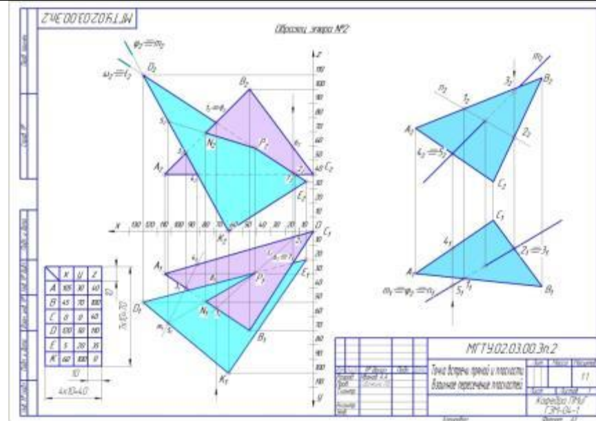
Эпюра 3 «Сечение поверхности плоскостью. Натуральная величина сечения»
