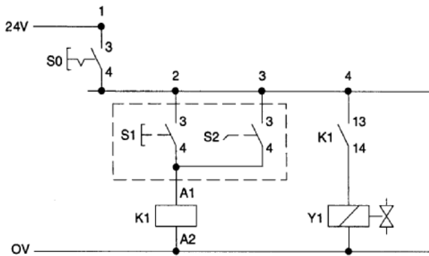
2 электрическая схема
