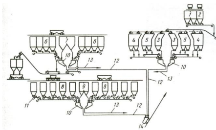
Рис. 6. Схема шихтоподдачи доменной печи "Аманда" объемом 2032 м 3 . 1 – бункера окатышей; 2, 3 – бункера известняка; 4 – бункера агломерата и руды; 5 – бункера окатышей и руды; 6, 7 – бункера кокса; 8 – бункера лобовок; 9 – бункер скрепы; 10 – весовые воронки; 11–13 – ленточные весы; 14 – склип
