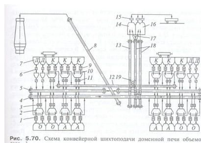
Рис. 5.70. Схема конвейерной шихтоподдачи доменной печи объемом 5000 м 3
