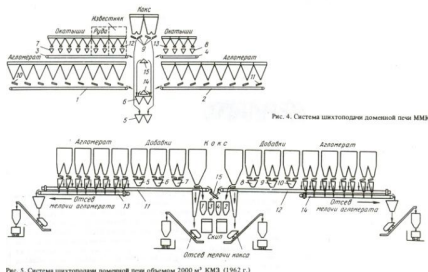
Рис. 5. Система шихтоподдачи доменной печи объемом 2000 м 3 КМЗ (1962 г.)
