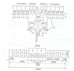
Рис. 5.69. Схема транспортной шихтоподдачи к склякам доменной печи объемом 1200 м³. 1 – гранулы агломерата; 2 – конвейер агломерата; 3 – перекидной ящик; 4, 6, 10 – конвейер кокса; 5 – конвейер кокса; 7 – конвейер кокса; 8 – конвейер кокса; 9 – гранулы кокса; 11 – конвейер кокса мелкого.
