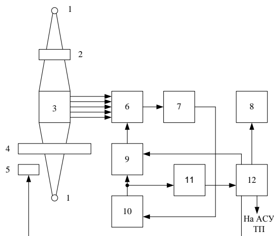
1 – источник излучения; 2 – образцы толщин; 3 – сцинтилляционный кристалл; 4 – объект контроля в виде полосы; 5 – подвижный образец толщины; 6 – фотоэлектронный умножитель (ФЭУ); 7 – усилитель; 8 – показывающий прибор; 9 – блок питания ФЭУ; 10 – регулятор тока ФЭУ; 11 – блок обработки сигнала; 12 - контроллер Рисунок 1 – Структурная схема рентгеновского толщиномера
