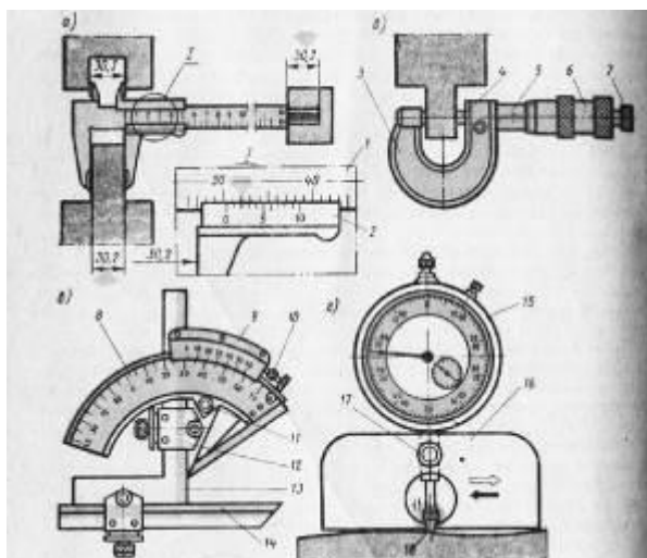
Рис. 1. Инструменты: а — щуп, б — брусовый уровень, в - рамный уровень, г — приспособления для проиндикатор, д — магнитная стойка, е — контрольная оправка, верки точности станков: ж — контрольный диск; 1 — пузырек воздуха, 2 — ампула, 3 — указатель оборотов, 4 — измерительный наконечник, 5 — циферблат, 6 — стрелка, 7 — основание, 8 — штатив, 9 — индикатор, 10 — винт, 11 — конический хвостовик, 12 — цилиндрическая часть
