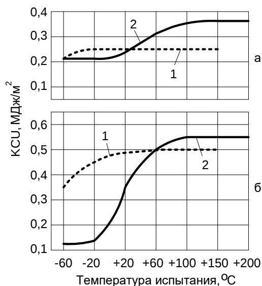
Рис. Вязкость сталей 6XC (1) и 6XB2C (2) в зависимости от температуры испытания:
