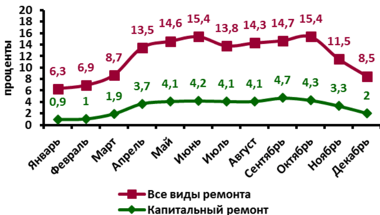
Динамика изменения ремонтной мощности ТЭС, ГЭС и АЭС ЕЭС России в 2017 году
