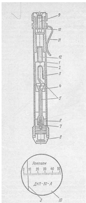
Рис. 4 Дозиметр карманный прямопоказывающий ДКП-50А 1 – окуляр; 2 – шкала; 3 – дюралевый цилиндрический корпус; 4 – подвижная платинированная нить; 5 – внутренний электрод (алюминиевый стержень); 6 – конденсатор; 7 – защитная оправа; 8 – защитное стекло; 9 – ионизационная камера; 10 – объектив; 11 – держатель; 12 – фасонная гайка
