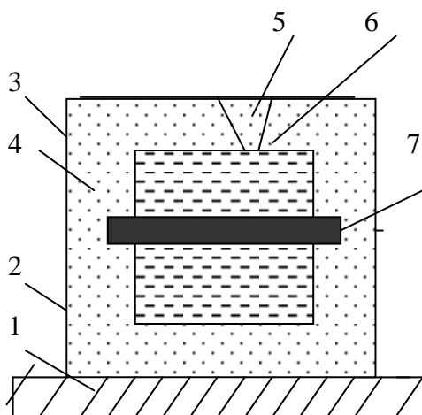
Рис. 1. Литейная форма
