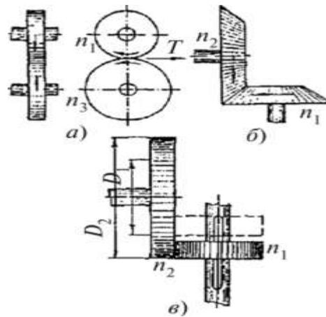
Рис. 11.2. Фрикционные передачи с цилиндрическими (а) и коническими (б) колесами и торцовый вариатор (в)
