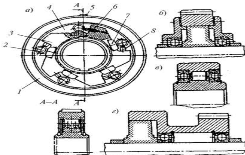
Рис. 11.4. Фрикционная обгонная муфта {а), установка подшипников
