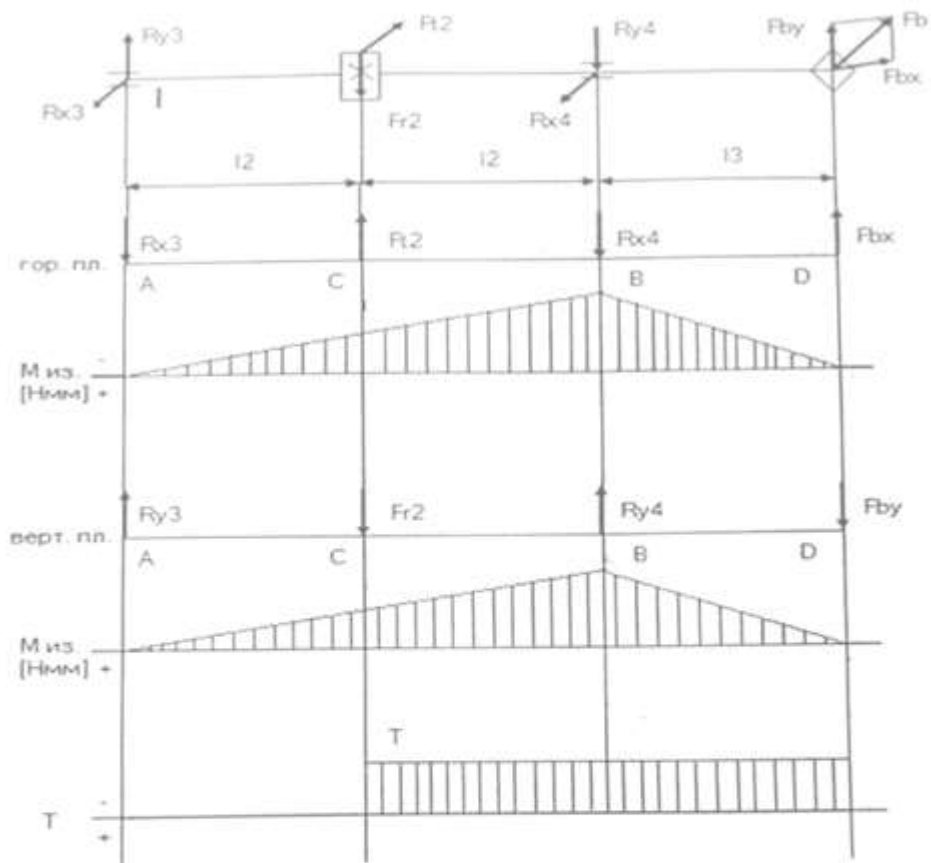
Рисунок 6 – Ведущий вал.
