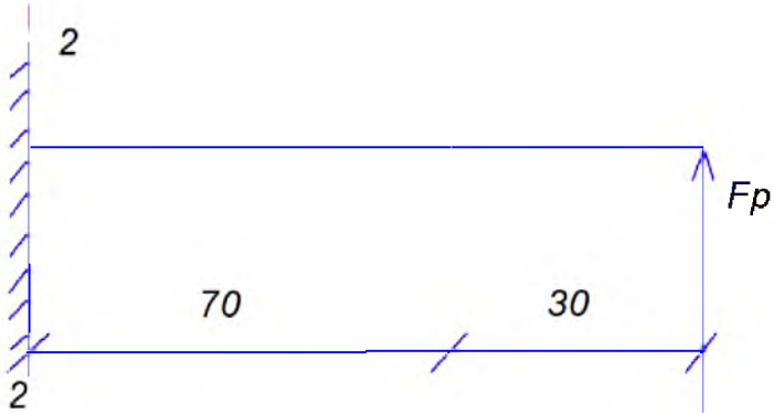
Рисунок-6 График расчета вилка на поперечный изгиб Изгибающий момент в сечении 1.1.
