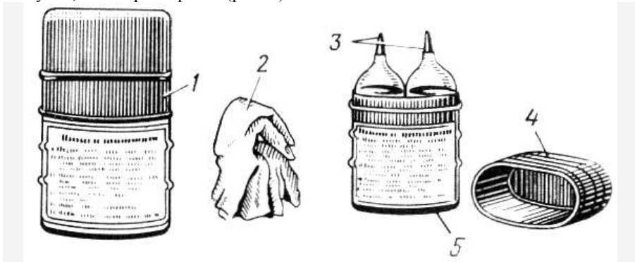
Рис. 4. Индивидуальный противохимический пакет ИПП-8 (1 – жестяной фужляр; 2 – бумажные салфетки; 3 – стеклянные ампулы; 4 – крышка; 5 – памятка по пользованию пакетом)
