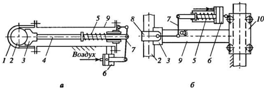
Рисунок 4 — Схема электрододержателей
