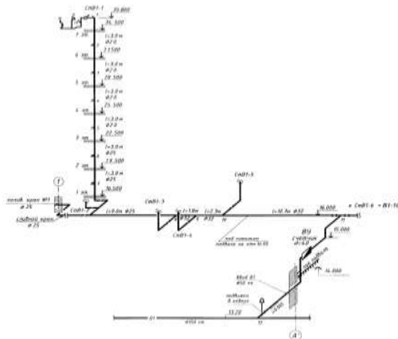
Рис. 4. Аксонометрическая схема холодного водопровода
