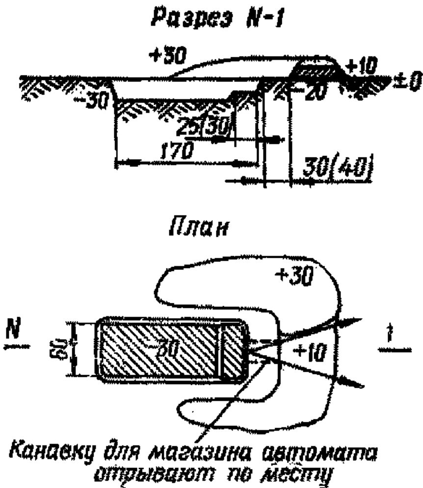
Рис.5 Одиночный окоп для стрельбы из автомата лежа
