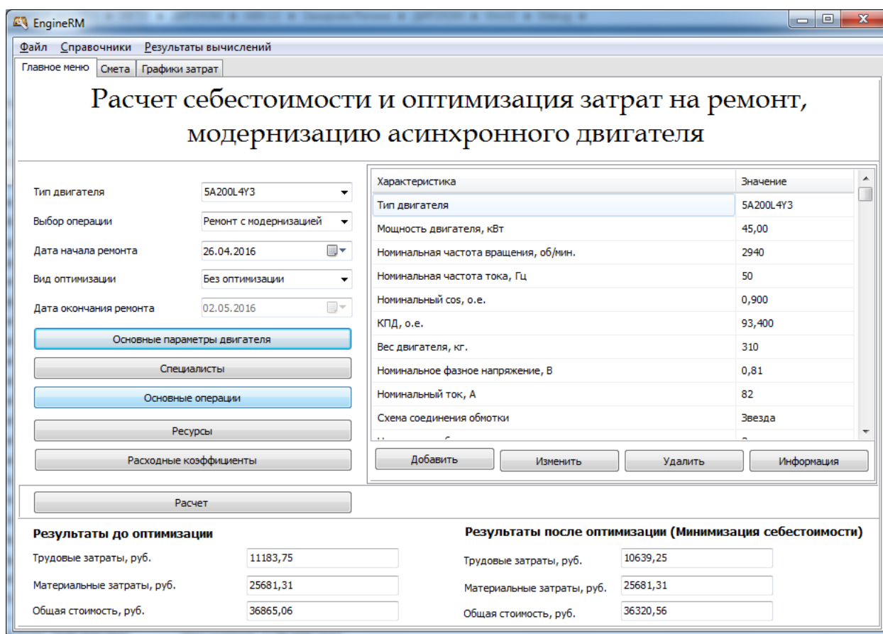
Рисунок 1 – Рабочее окно программы
