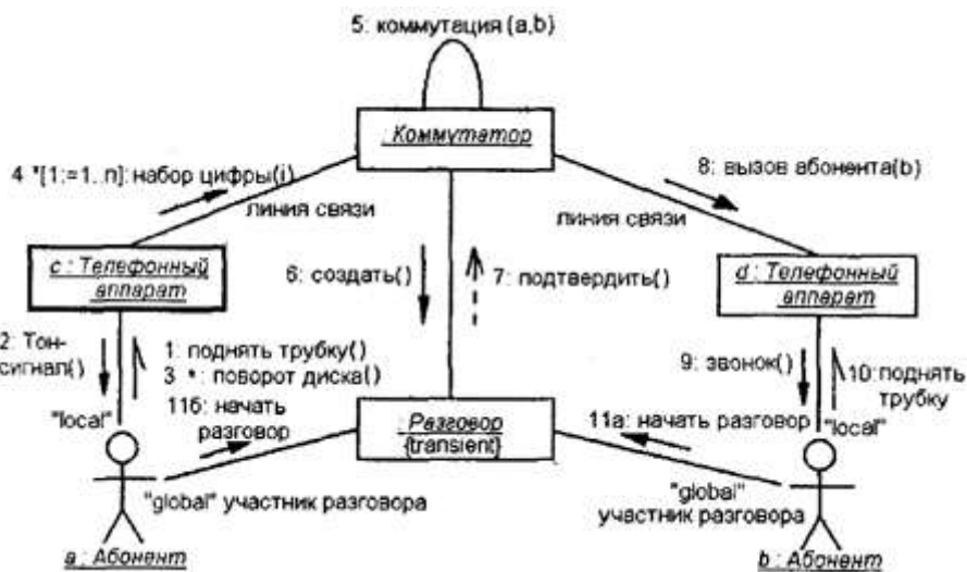
Рис. 10. Окончательный вариант диаграммы кооперации для моделирования телефонного разговора
