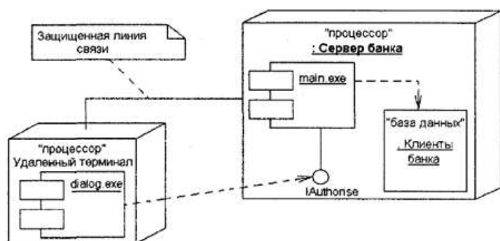
Рис. 5. Диаграмма развертывания для системы удаленного обслуживания клиентов банка
