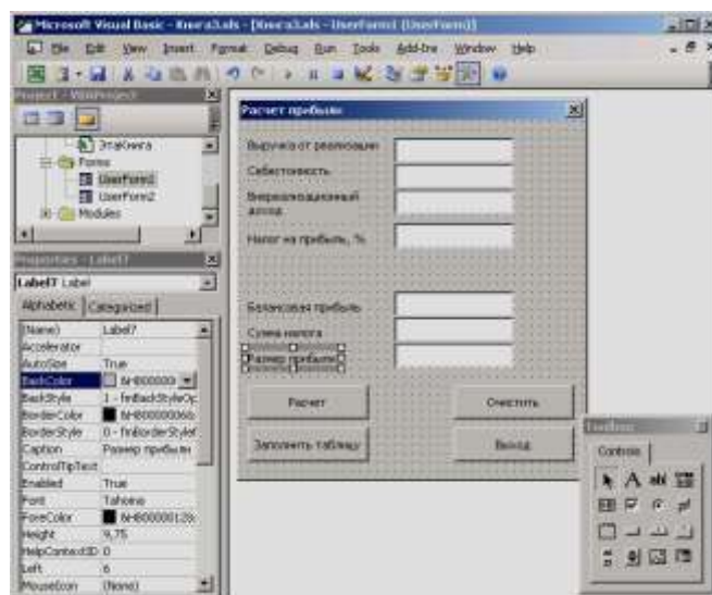
Рис. 19. Форма «Расчет прибыли» в окне редактора VB
