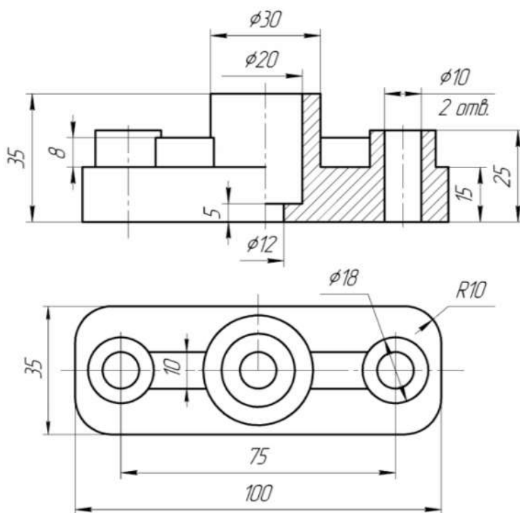
Рисунок 1 – Чертеж детали «Опора»
