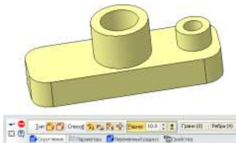
Рисунок 26 – Скругление ребер основания радиусом 10 мм
