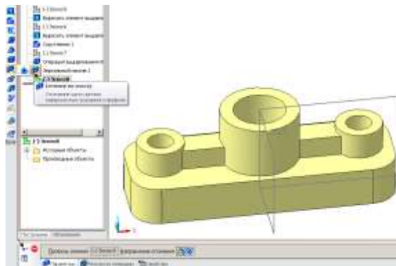
Рисунок 36 – Вид эскиза сечения в системе трехмерных построений
