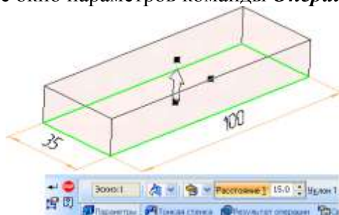
Рисунок 6 – Диалоговое окно параметров команды Операция выдавливания
