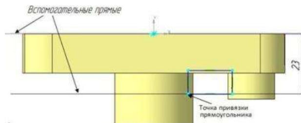
Рисунок 28 – Эскиз ребра жесткости
