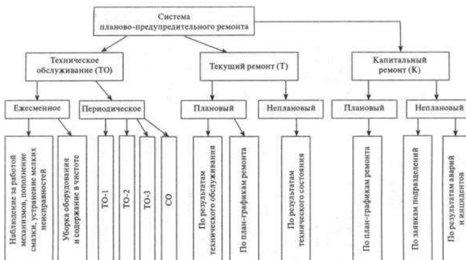
Рис.2 Система планово-предупредительного ремонта
