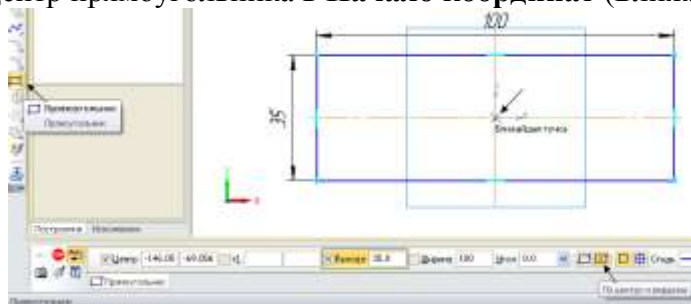
Рисунок 4 – Построение контура основания с помощью команды Прямоугольник
