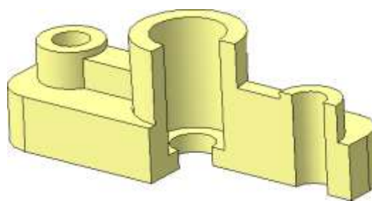
Рисунок 37 – Усеченная модель «Опора»
